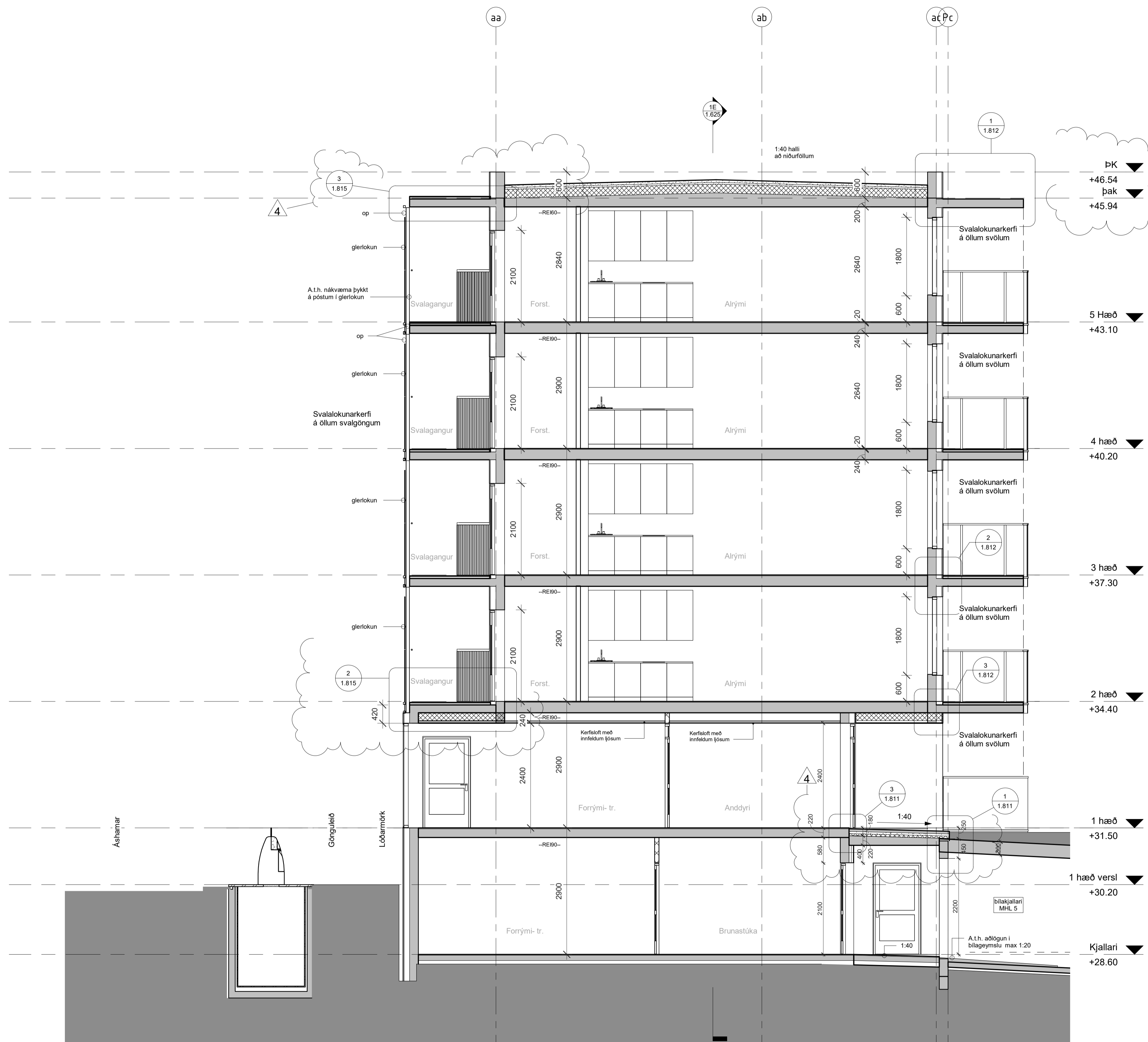
C-C inngangur 1:50
