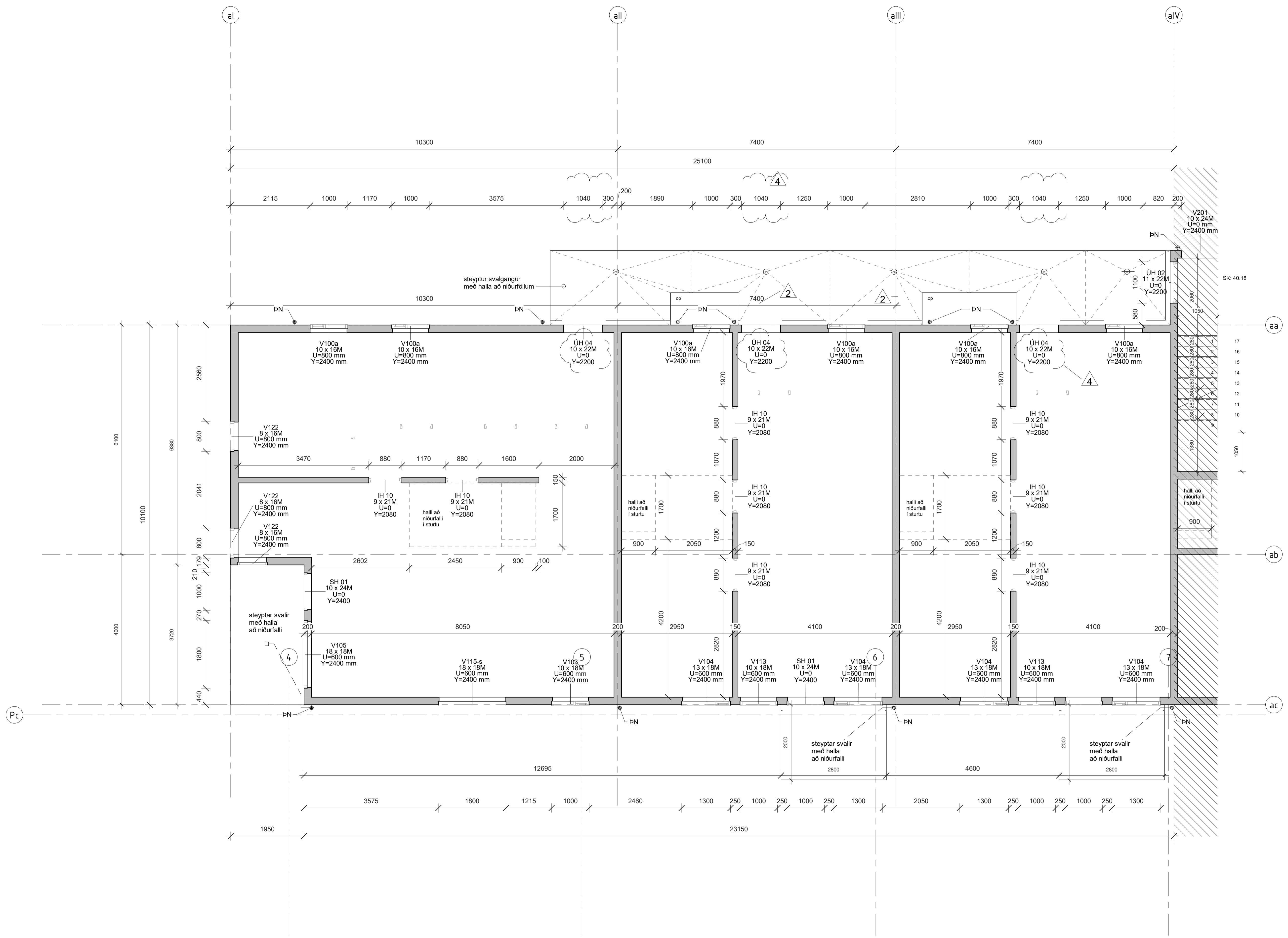
4 hæð-Steypa - sl 1 : 50
