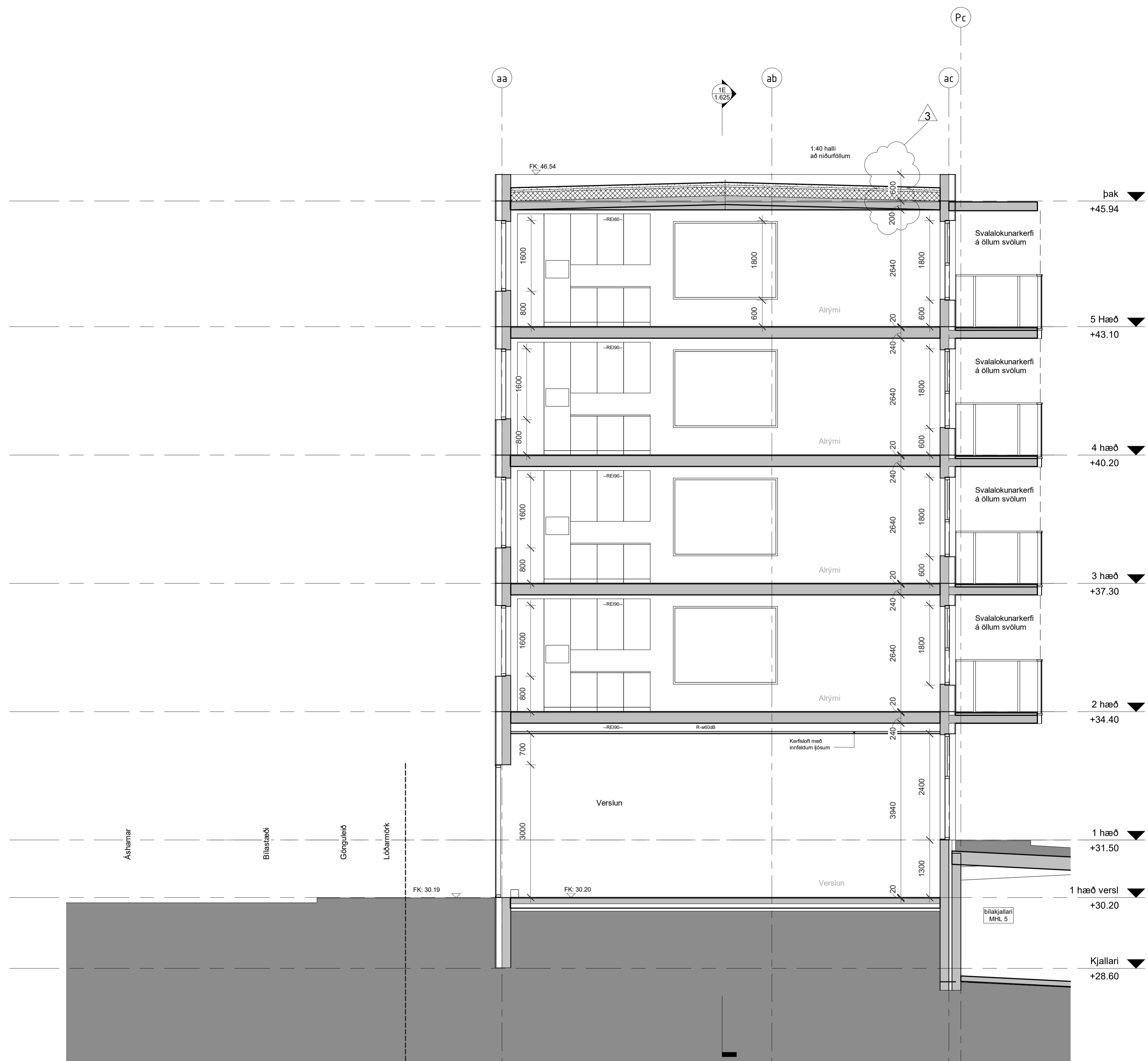
D-D verslun vt 1:50
