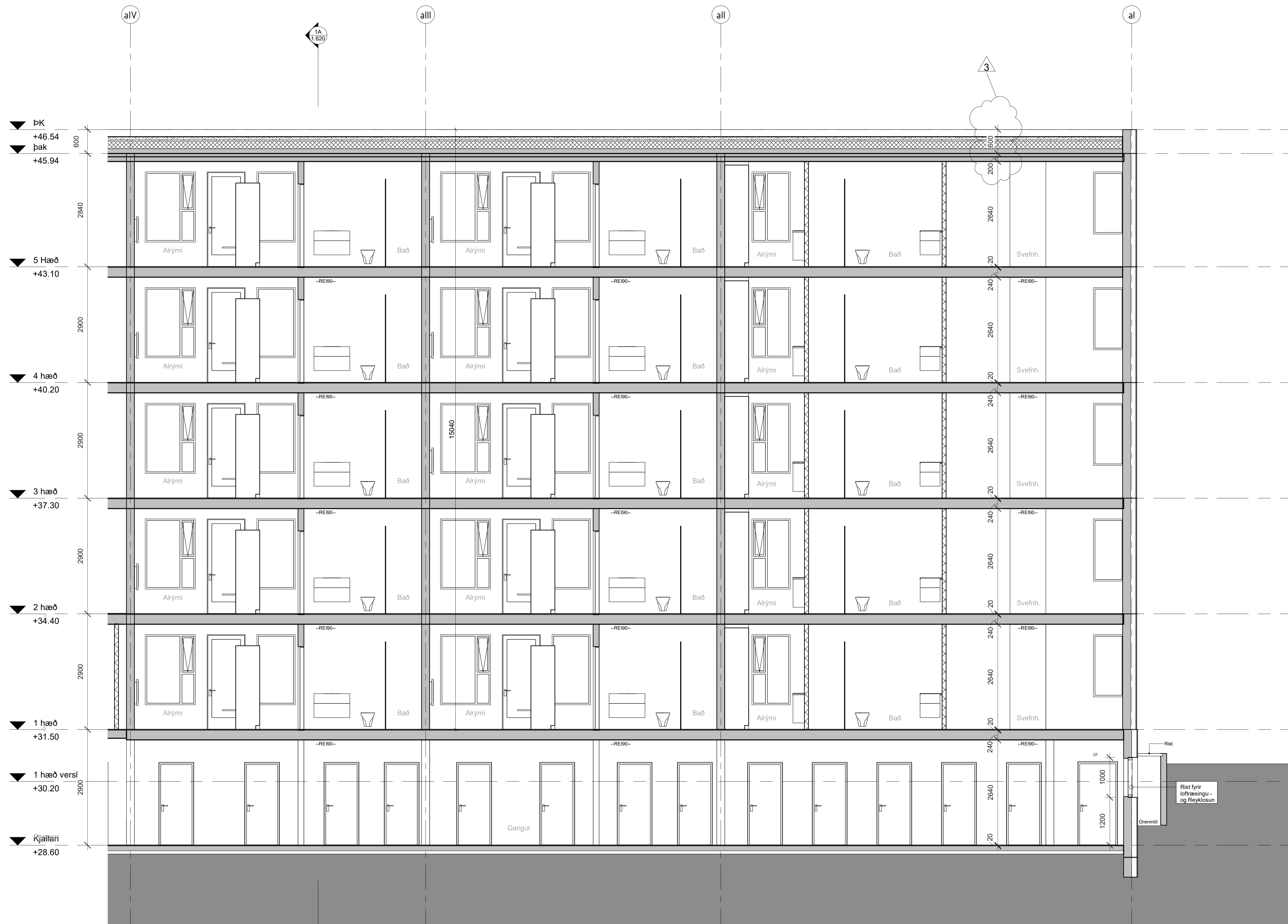
E-E langsníð 1 vt 1 : 50
