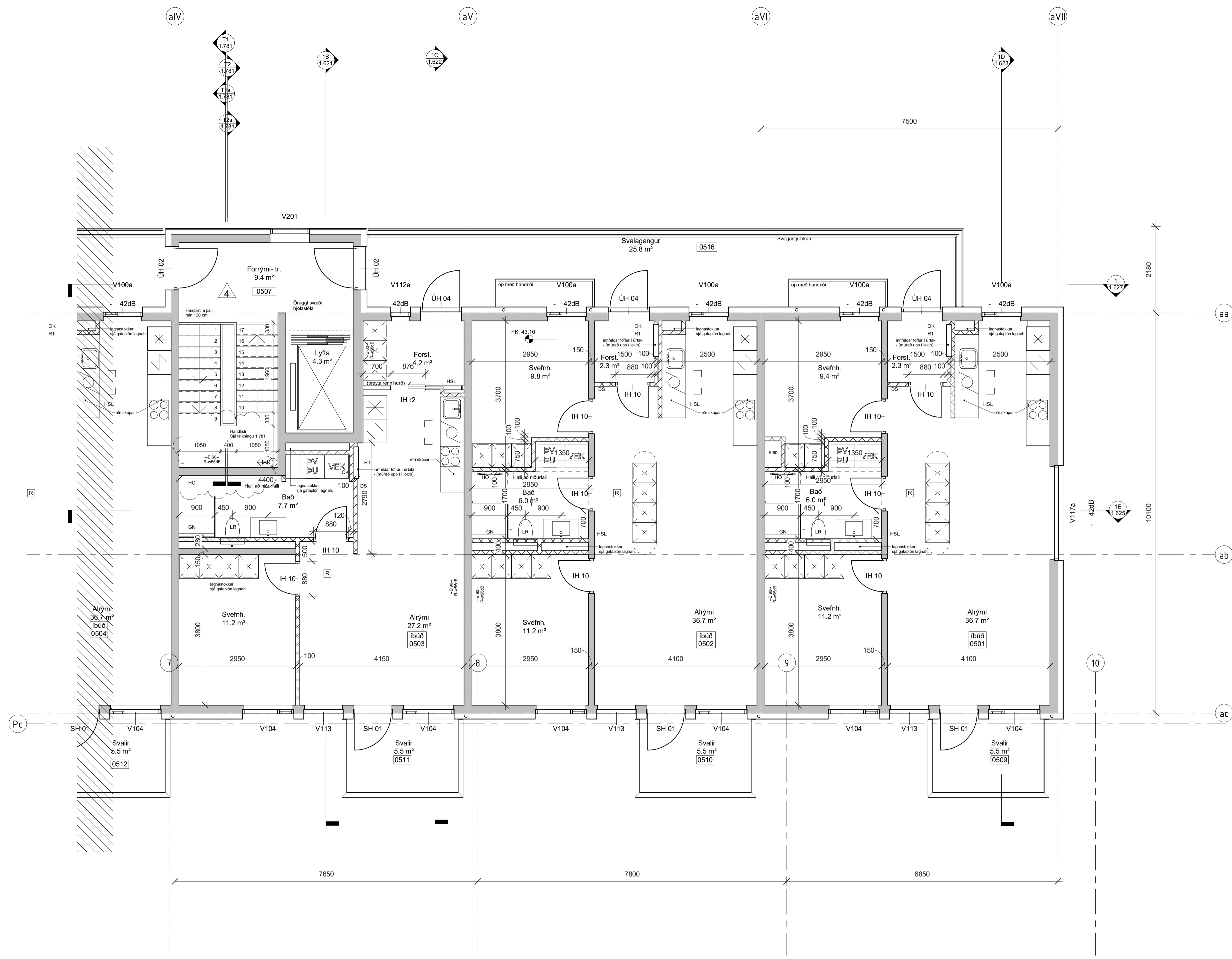
5 Hæð-vt - sll 1 : 50
