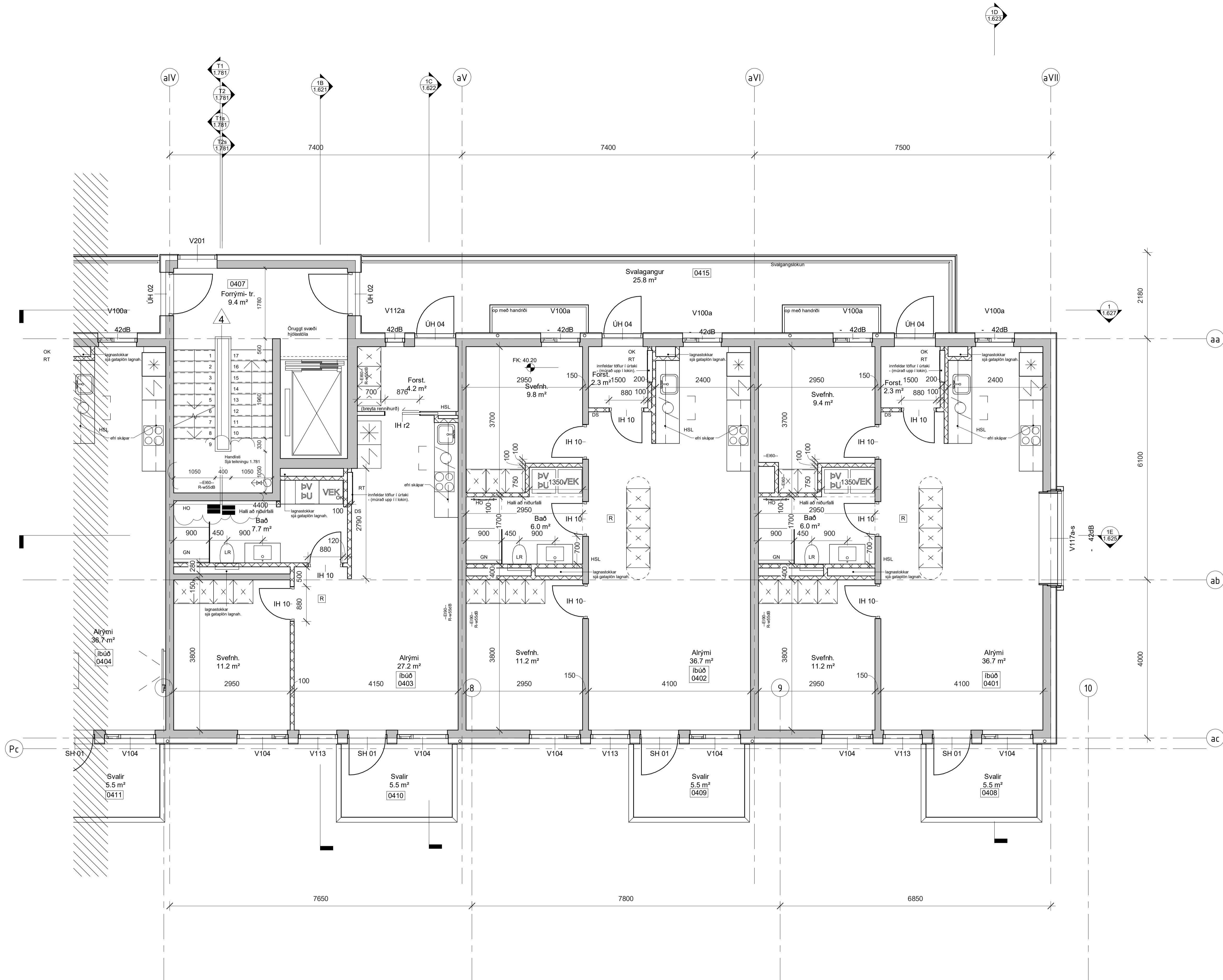
4 hæð-vt - sll 1:50
